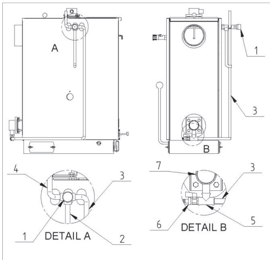
obr. 3. Připojení DBV 1 ke kotlům VARIANT
