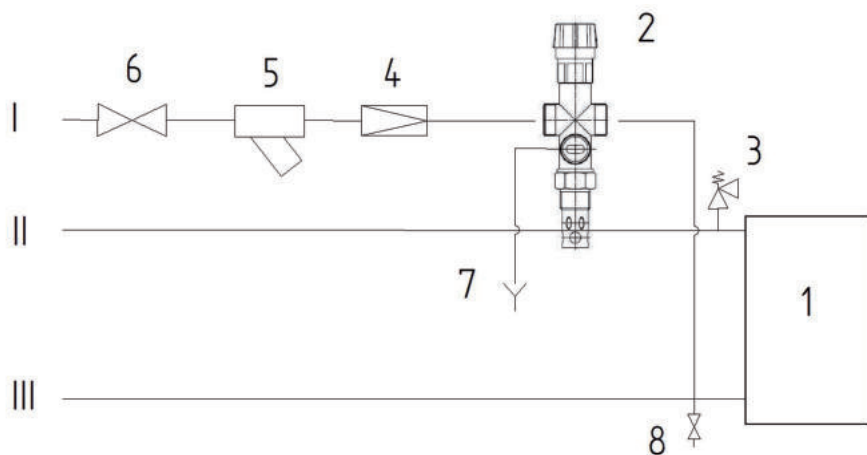
obr. č. 4 Schéma zapojení DBV 1
