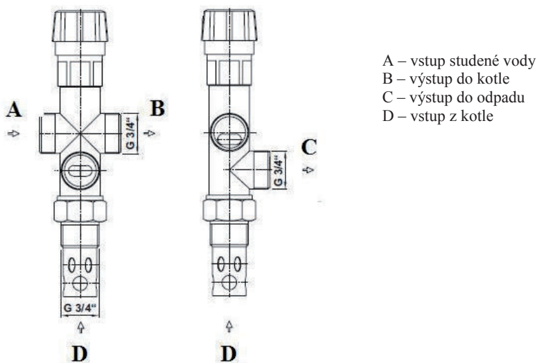
obr. 3 Dvoucestný bezpečnostní ventil DBV 1
